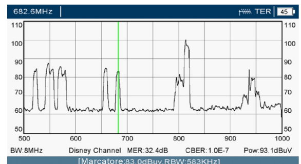
Fig. 19 Misura segnali 2G e 4G (si vedono i canali di downlink assieme ai canali DVB-T)
