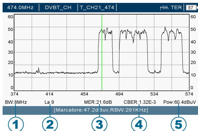
Fig. 10 Spettro segnali digitali terrestri
