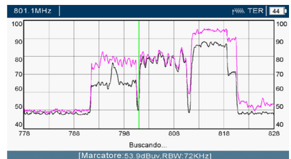
Fig. 18 Misura di un segnale interferente 4G (canali di downlink)
