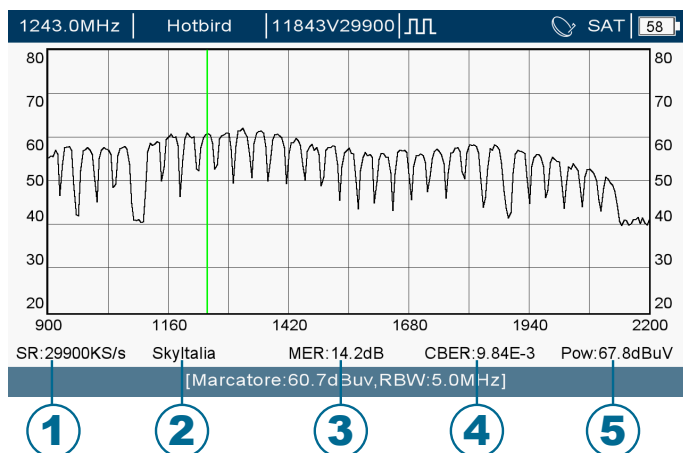
Fig. 9 Spettro segnali satellitari
