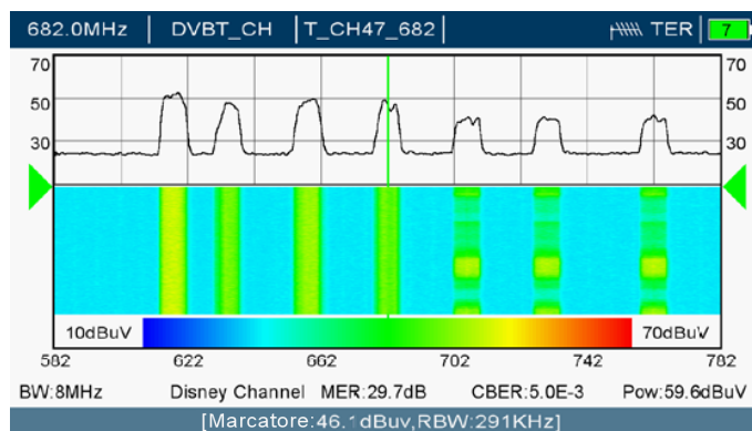
Fig. 15 Effetto di un fading, dove i tre canali alti soffrono variazioni di livello del loro segnale
