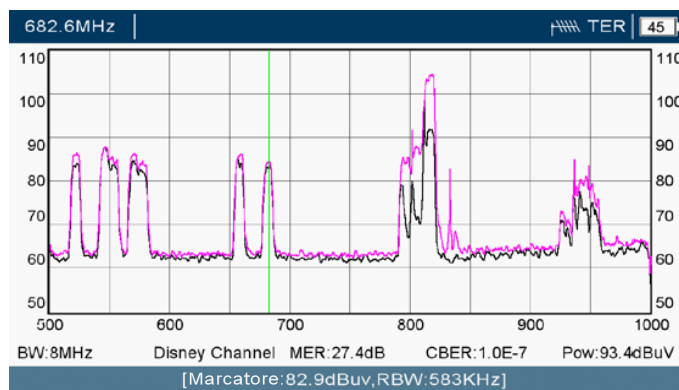
Fig. 16 Immagine con sette mux DTT e picchi massimi della telefonia mobile 3G/4G.
