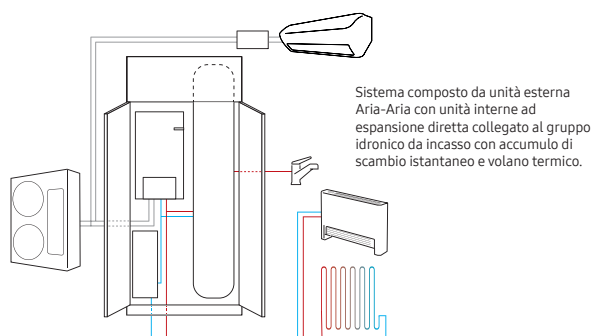
EHS TDM PLUS + Unità Interne + Gruppo idronico da incasso + Volano termico
