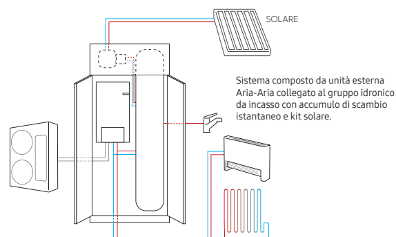
EHS SPLIT + Gruppo idronico da incasso + Kit Solare
